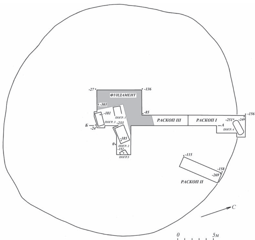
Рис. 2. Мавзолей № 1 у пос. Красный. План расположения раскопов
