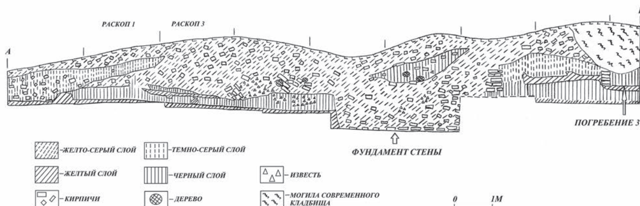
Рис. 4. Мавзолей № 1 у пос. Красный. Профиль по линии А–Б
