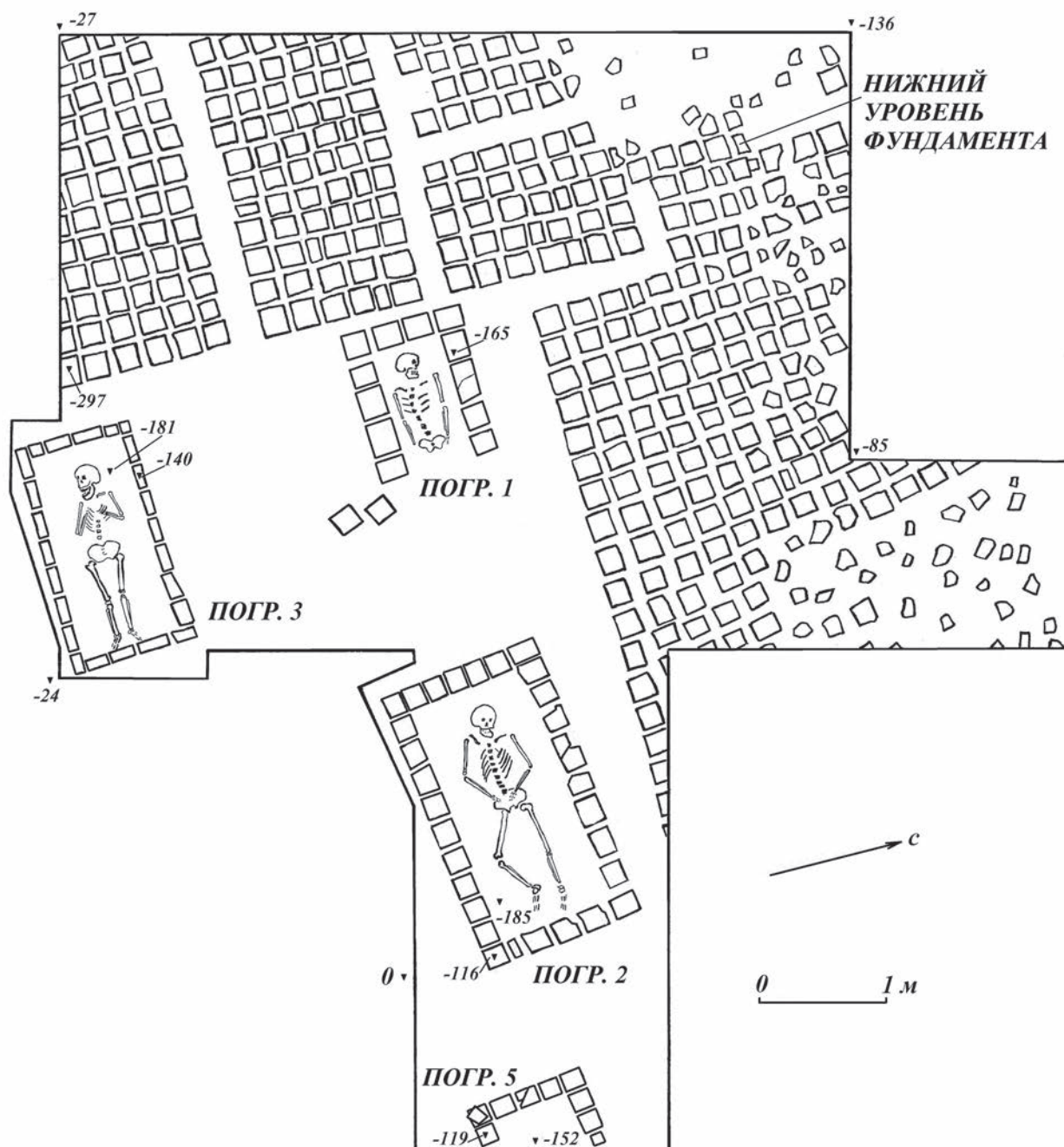
Рис. 3. Мавзолей № 1 у пос. Красный. План раскопа III
