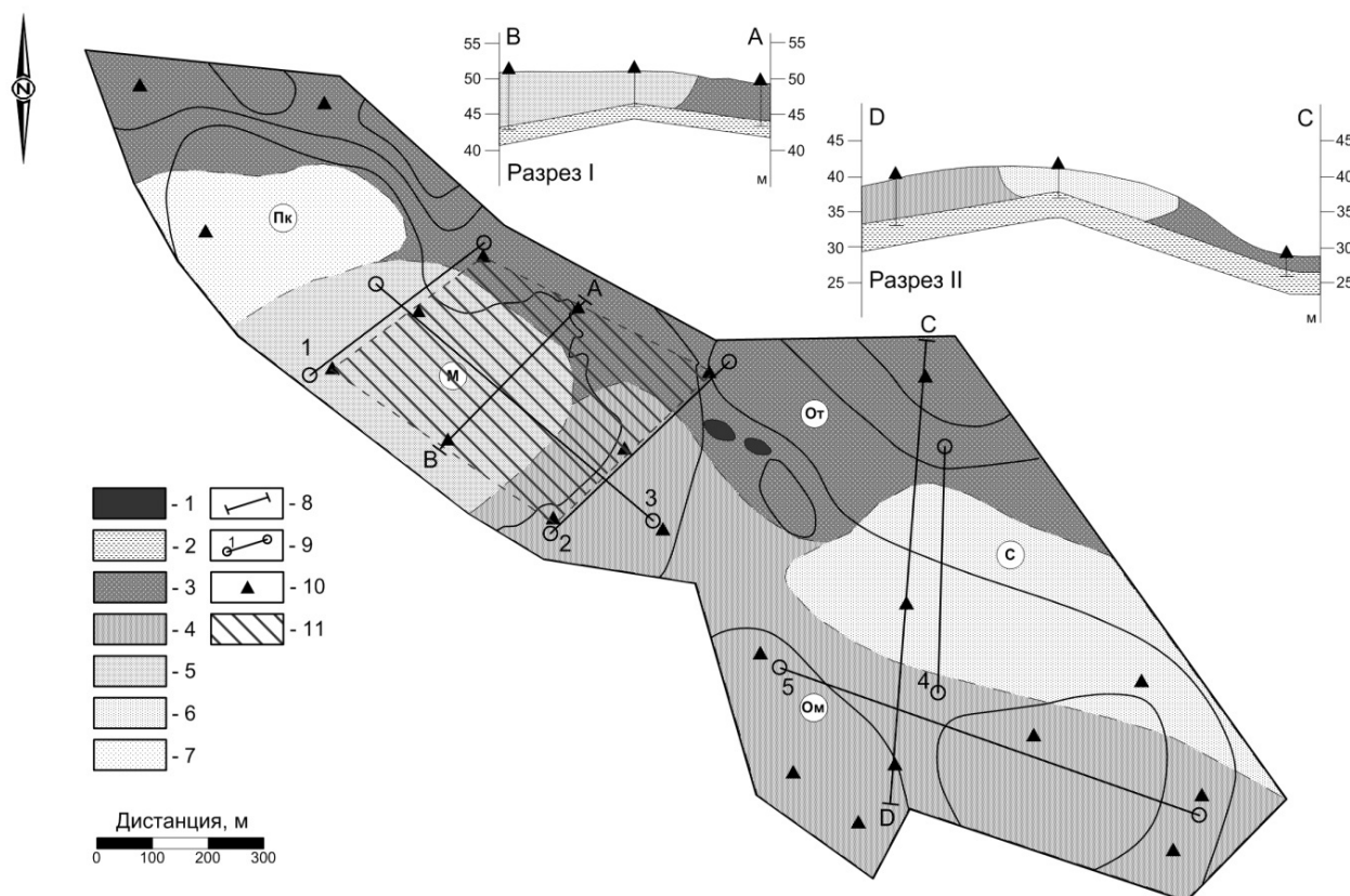
Рис. 3 Геологическая схема исследуемого месторождения (с разделением песка по крупности согласно ГОСТ 8736-93): 1 – дочетвертичные образования; 2 – супесь; 3 – песок очень тонкий; 4 – песок очень мелкий; 5 – песок мелкий; 6 – песок средний; 7 – песок повышенной крупности; 8 – геологические разрезы; 9 – профиль георадиолокации и его номер; 10 – скважины; 11 – блок подсчета запасов по категории С 1 .
