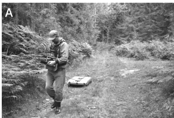
Рис. 1 Фотографии георадарной съёмки в полевых условиях: А – процесс съёмки; Б – анализ радарограммы в полевых условиях.
