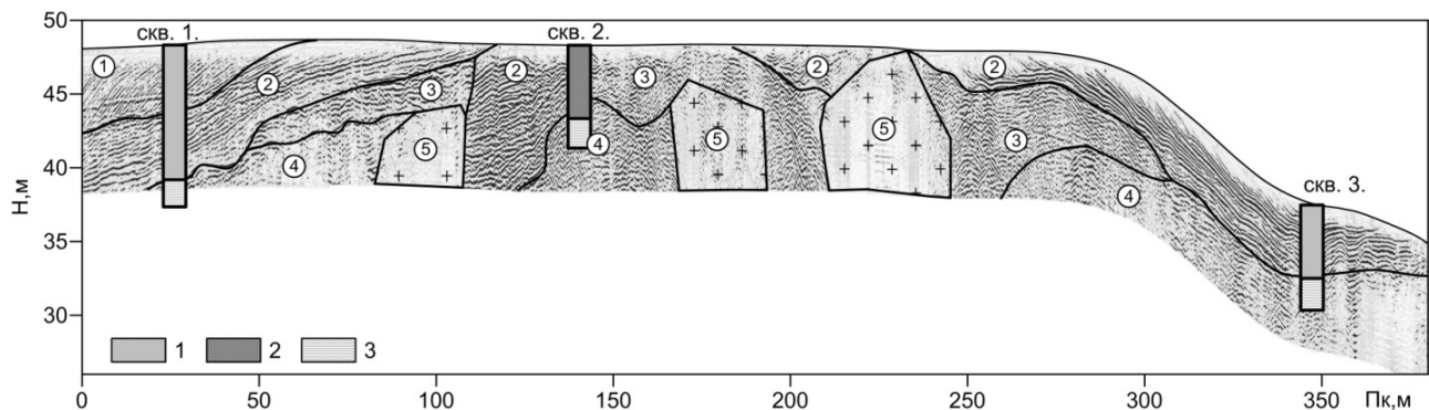
Рис. 6 Георадарный профиль № 2: 1 – пески наклонного залегания; 2 – пески косого залегания; 3 – пески с включением гальки и гравия; 4 – суглинки; 5 – коренные породы. Легенда для буровых колонок: 1 – тонкозернистый песок; 2 – мелкозернистый песок с галькой; 3 – суглинок.
