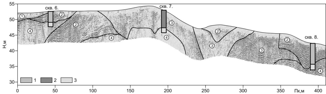
Рис. 5 Георадарный профиль № 1: 1 – пески наклонного залегания; 2 – пески косого залегания; 3 – пески с включением гальки и гравия; 4 – суглинки. Легенда для буровых колонок: 1 – тонкозернистый песок; 2 – мелкозернистый песок с галькой; 3 – суглинок.
