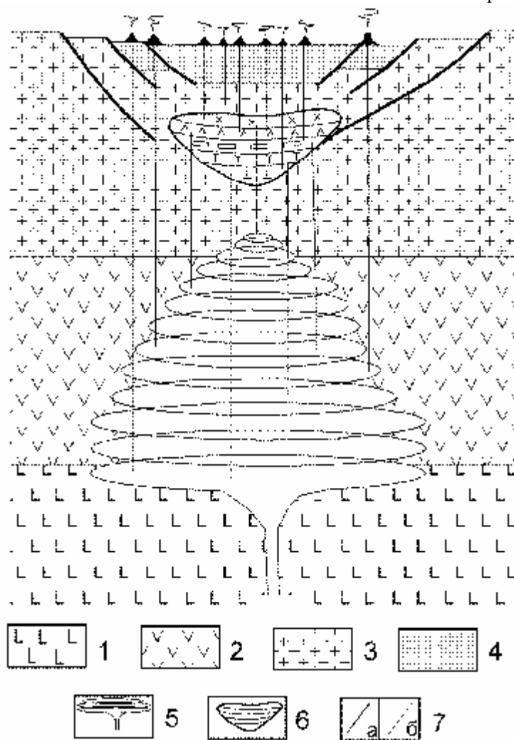
Рис. 5. Предполагаемый механизм формирования расплавов кремнеземистой высокомагнезиальной (бонинитоподобной) серии
