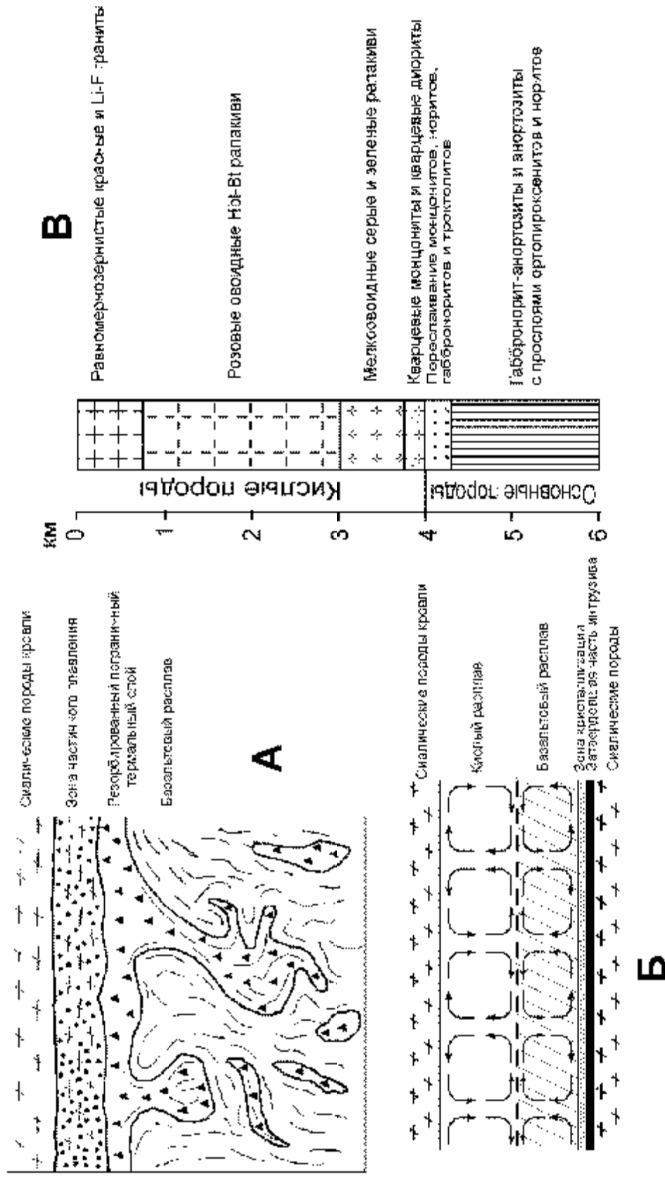
Рис. 2. Схемы, иллюстрирующие процессы в кровле мощного базитового силла и строение итогового тела: а - начальные стадии процесса; б - развитые стадии процесса (по [20], модифицирована автором); в - строение итогового тела в магматической системе АРГК
