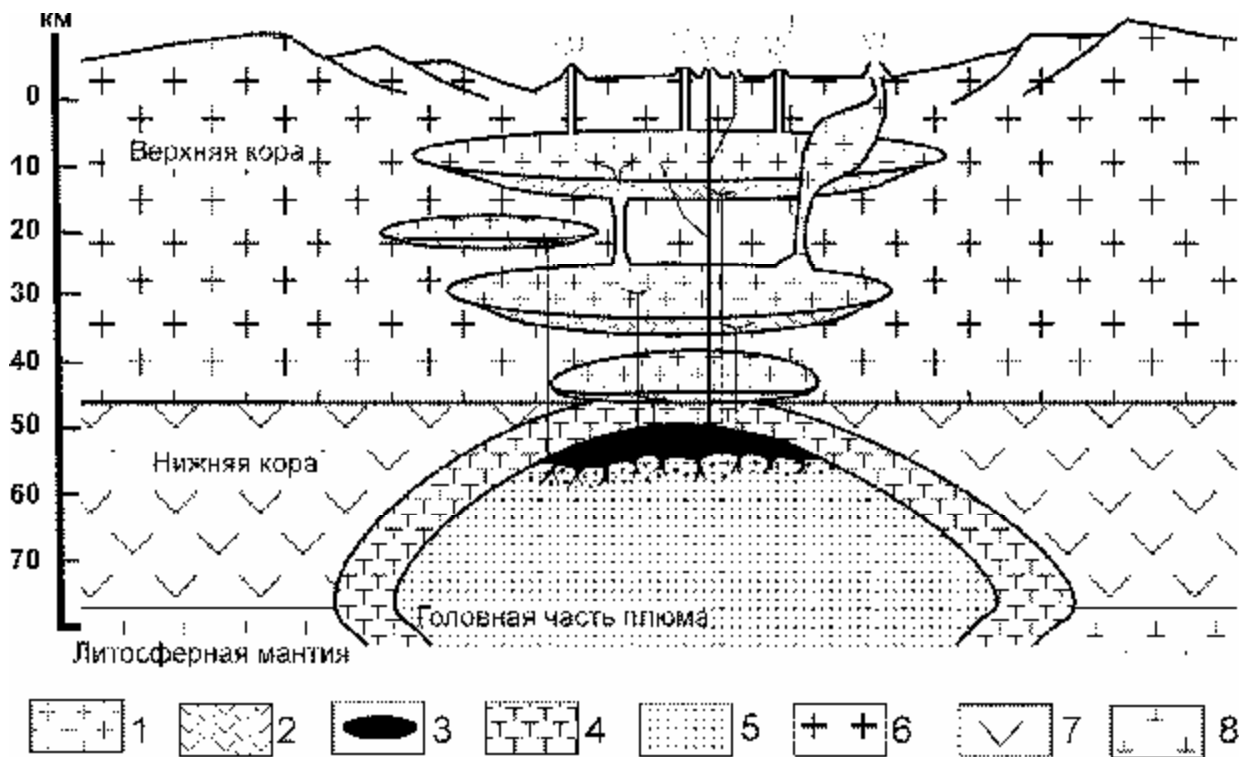
Рис. 3. Принципиальная схема строения транскоровой магматической системы, возникшей над локальным плюмом в условиях anomalно мощной коры при формировании анортозит-рапакиви-гранитных комплексов: 1 - гранитный расплав и продукты его затвердевания; 2 - базитовый расплав и продукты его затвердевания; 3 - область мантийного магнезиального образования; 4-5 - головная часть плюма; 4 - его охладившаяся краевая зона, 5 - внутренняя часть плюма; 6 - древняя сиалическая кора; 7 - древняя нижняя базитовая кора; 8 - древняя литосферная мантия
