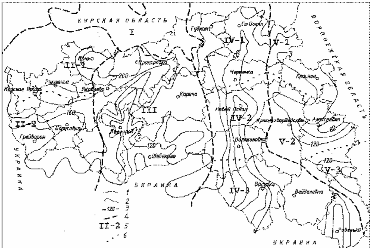
Рис. 2. Схема гидрогеологических подрайонов: 1- административные границы Белгородской области; 2 - административные границы районов Белгородской области; 3 – гидроизогипы нижнемелового водоносного комплекса; 4 – границы гидрогеологических районов; 5 – индекс гидрогеологического подрайона; 6 – граница гидрогеологического подрайона
