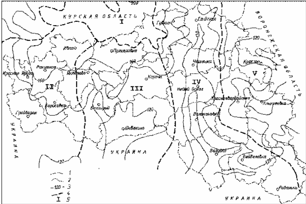
Рис. 1. Схема гидрогеологических районов: 1- административные границы Белгородской области; 2 - административные границы районов Белгородской области; 3 – гидроизогипы верхнемелового водоносного комплекса; 4 – границы гидрогеологических районов; 5 – индекс гидрогеологического района
