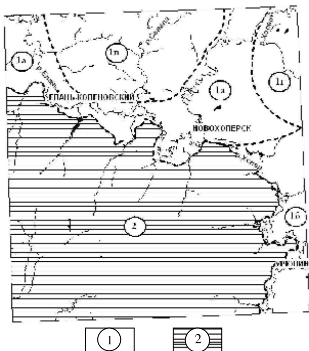
Рис. 1. Схема неотектонической структуры территории листа М-37-ХП: 1 - Окско-Донская впадина (1а – Масальский неотектонический прогиб; 1б Урюпинский неотектонический прогиб; 1в – Шукавкинское неотектоническое поднятие; 1г – Мучкапский неотектонический прогиб); 2 - Калачское поднятие
