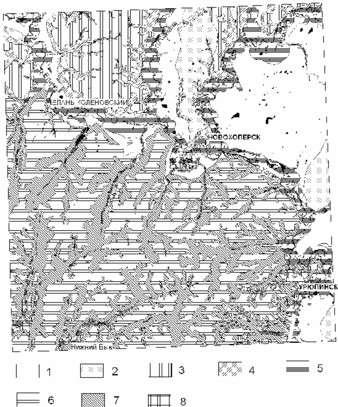
Рис. 2. Схема районирования условий развития ЭГП на территории листа М-37-ХП масштаба 1:500 000: 1 – 8 номера районов (названия районов приведены в тексте)
