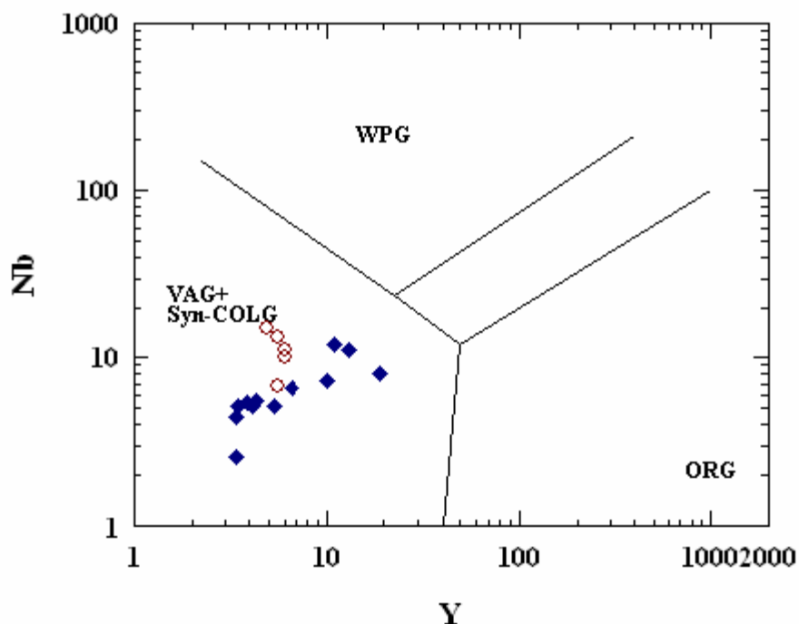
Рис. 6. Положение гранитоидов заганского и витимканского комплексов на бинарной диаграмме Y-Nb (основа графики по [16]). Поля на диаграммах : syn-COLG – синколлизии, WPG – внутриплитные, VAG – гранитоиды островных дуг, ORG- океанического дна. Условные обозначения: ○ -породы заганского комплекса, ◆ - породы витимканского комплекса
