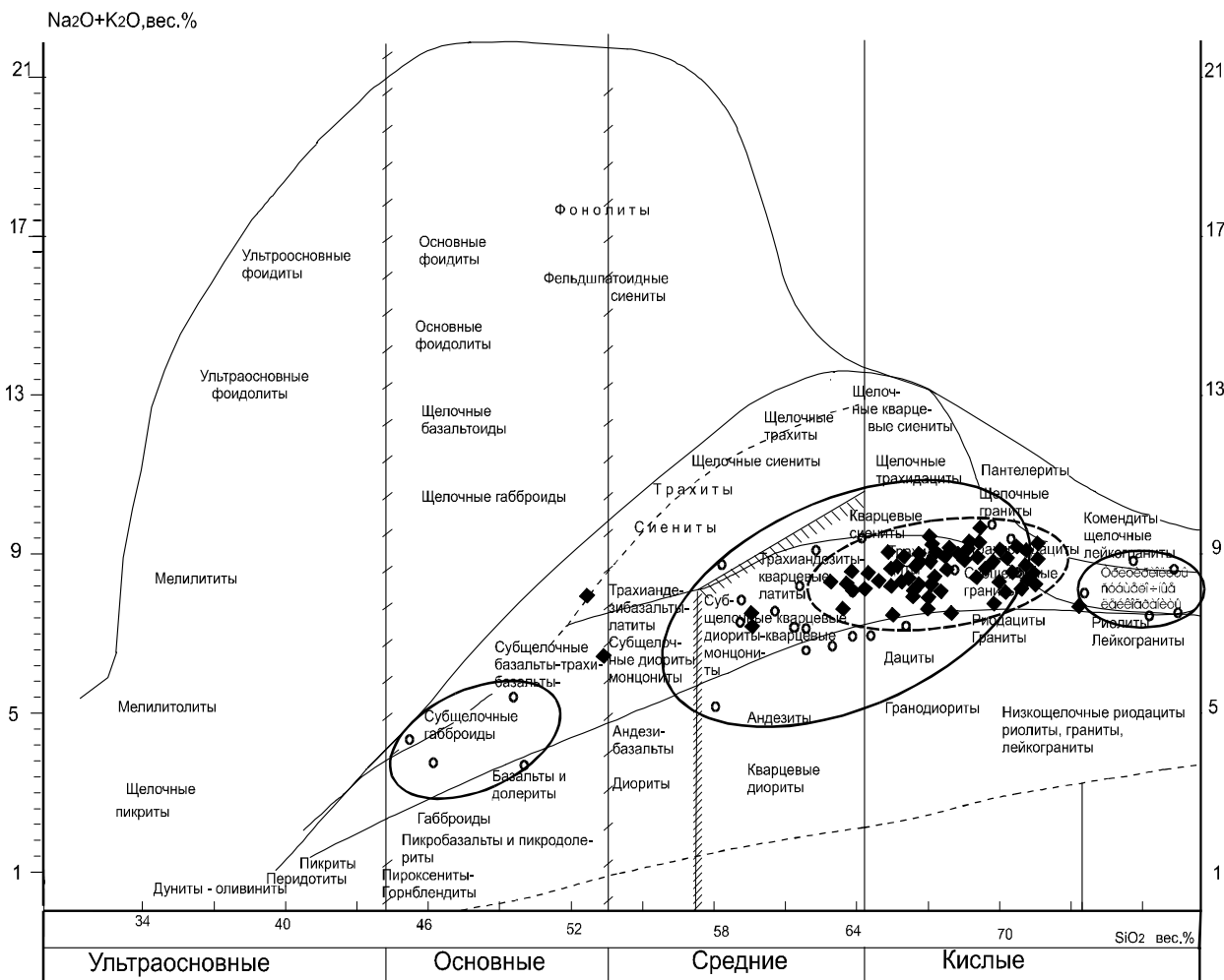
Рис. 2. Классификационная диаграмма (основа графики по [10]) для пород заганского и витимканского комплексов. Условные обозначения: \odot - результаты химического анализа пород заганского комплекса, \blacklozenge - результаты химического анализа пород витимканского комплекса
