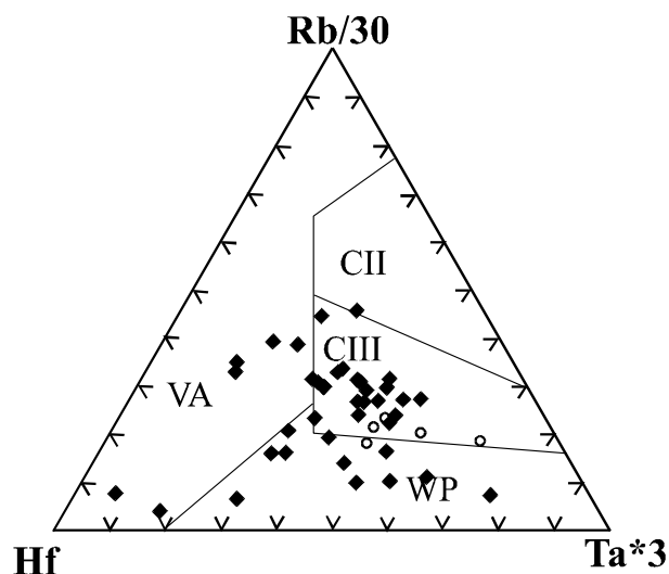
Рис. 8. Положение гранитоидов заганского и витимканского комплексов на тройной диаграмме Hf – Rb/30 – Ta*3 (основа графики по [17]). Поля на диаграммах : VA – островодужные; CII – коллизийные коровые; CIII – коллизийные подкоровые; WP – внутриплитные (анорогенные). Условные обозначения: ○ – породы заганского комплекса, ◆ – породы витимканского комплекса
