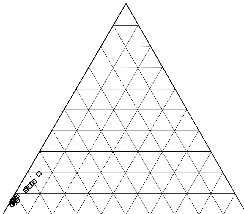
Рис. 3. Диаграмма \Sigma LREE (La-Nd) - \Sigma MREE (Sm-Ho) - \Sigma HREE (Er-Lu) (основа графики по [12]). Услов-
