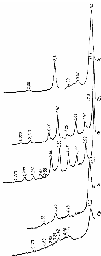
Рис. 1. Дифрактометрические кривые (фракция мельче 0, 001 мм) Na + – монтмориллонита из эоцена Асканы, Грузия: а - исходный образец, б – насыщенный этиленгликолем, в – насыщенный глицерином, г – обработанный 1 н. раствором КОН, д – обработанный насыщенным глицерином
