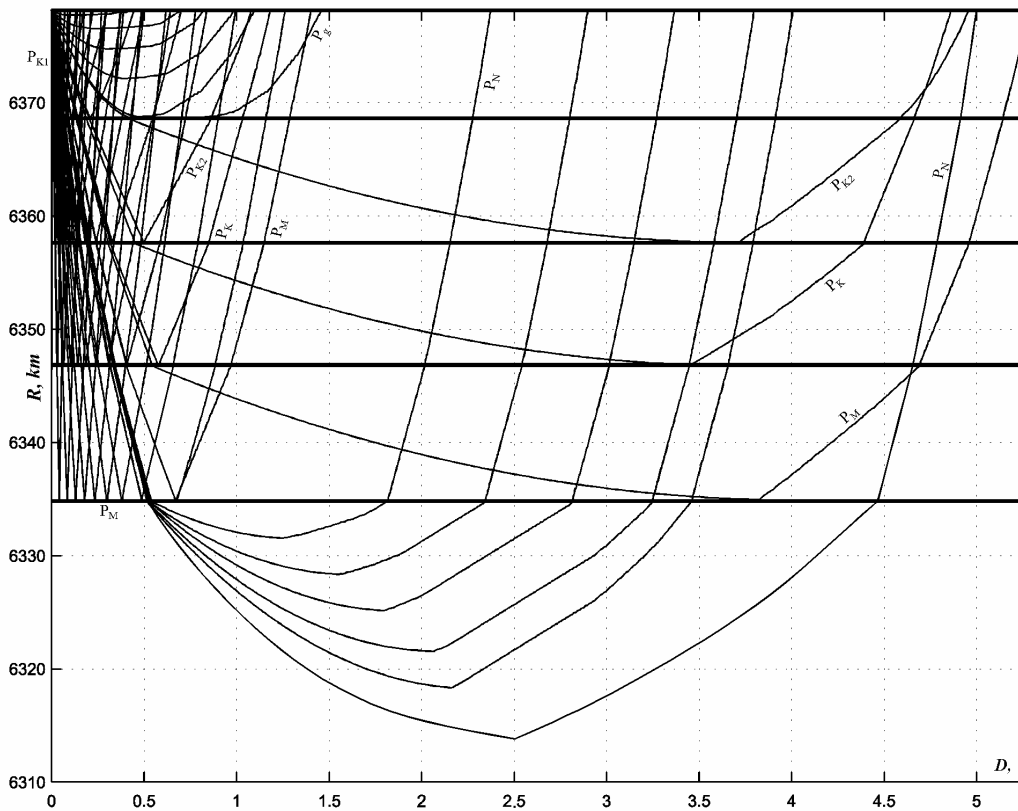
Рис. 2. Траектории лучей продольных волн для годографов, изображенных на рис. 1
