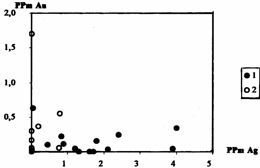
Рис. 11. Распределение золота и серебра в пиритах базальных конгломератов позднемелового (1) и девонского (2) возрастов Павловского карьера
