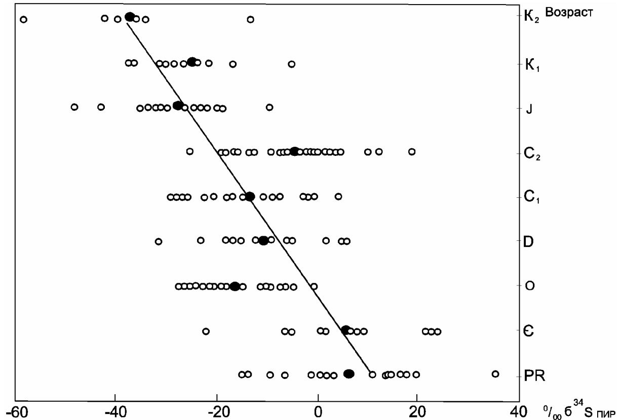
Рис. 8. Временной тренд изотопного состава серы в пиритах из разновозрастных отложений Воронежской антеклизы и других районов Русской платформы
