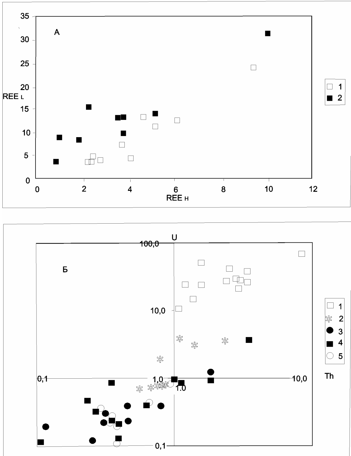
Рис. 9. Распределение редких земель, урана и тория в пиритах из разновозрастных пород Воронежской антеклизы: а – соотношение REE в пиритах базальных конгломератов позднемелового (1) и девонского (2) возрастов Павловского карьера; б – соотношения урана и тория в пиритах из верхнемеловых (1), нижнемеловых (2), юрских (3), девонских (4) и протерозойских (5) пород
