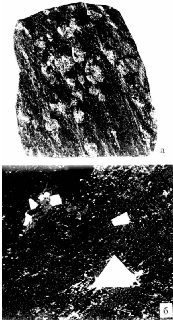
Рис. 5. Кубические кристаллы пирита (светлое) в железистом кварците: а – штуф, нат. величина; б – полир. шлиф, ув. 36,5. (Михайловский карьер)
