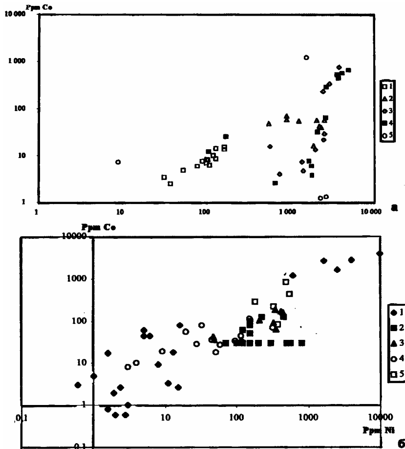
Рис. 10. Распределение кобальта и никеля в пиритах из разновозрастных пород Воронежской антеклизы (а) и других районов Русской платформы (б): а – пириты из пород позднемелового (1), раннемелового (2), юрского (3), девонского (4), протерозойского (5) возрастов; б – пириты из пород протерозойского (1 – Украинский щит, Рябоконец, 1983), девонского (2 – Припятская впадина, Михайлов, Каган, 1981), карбонового (3 – Донбасс, Кузнецов, Галий, 1984), кембрийского (4) и вендского (5 – Прибалтика, Битюкова, 1981) возрастов
