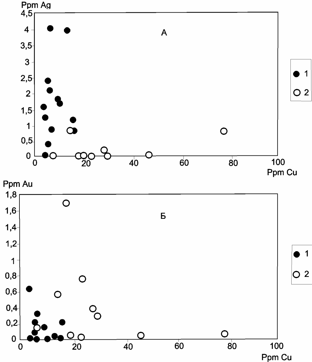
Рис. 12. Распределение серебра и меди (а), золота и меди (б) в пиритах базальных конгломератов позднемелового (1) и девонского (2) возрастов Павловского карьера
