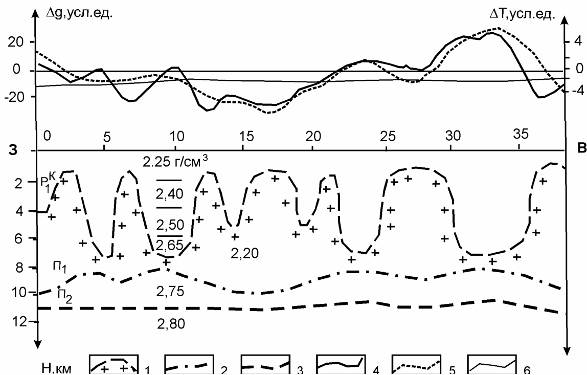
Рис. 3. Геолого-геофизическая модель по профилю 45 (по Е.Н. Волковой, Ю.П. Конценбину): 1 – поверхность соли P_1^K ; 2 – поверхность подсолевых отложений P_1 , связываемая с отражающим горизонтом \Pi_1 ; 3 – поверхность внутри палеозойских отложений, связываемая с отражающим горизонтом \Pi_2 ; 4 – наблюдаемая кривая \Delta g ; 5 – расчетная кривая \Delta g ; 6 – кривая магнитных аномалий \Delta T_a .
