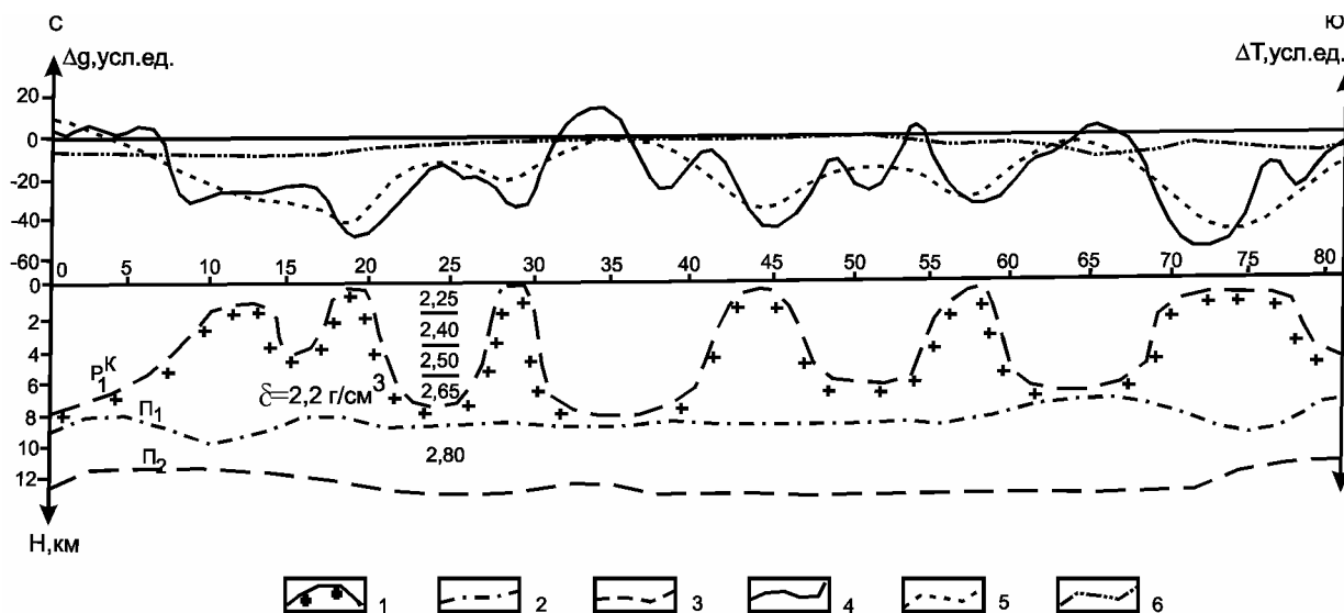
Рис. 4. Геолого-геофизическая модель по профилю 46 (по Е.Н. Волковой, Ю.П. Конценбину). Условные обозначения см. рис.3.
