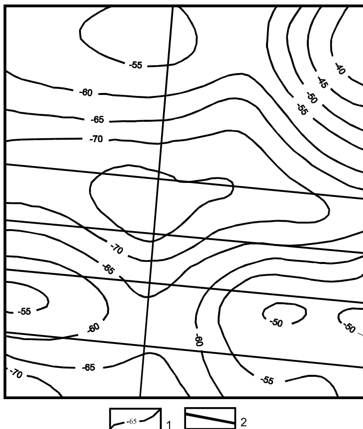
Рис. 2. Карта остаточных аномалий \Delta g_{\text{ост.}} = \Delta g_{\text{н}} - \Delta g_{\text{лок}} (по Е.Н.Волковой, Ю.П. Конценбину, Э.И. Столярову): 1 – изогравиметрические аномалии \Delta g , усл. ед.; 2 – расчетные профили.
