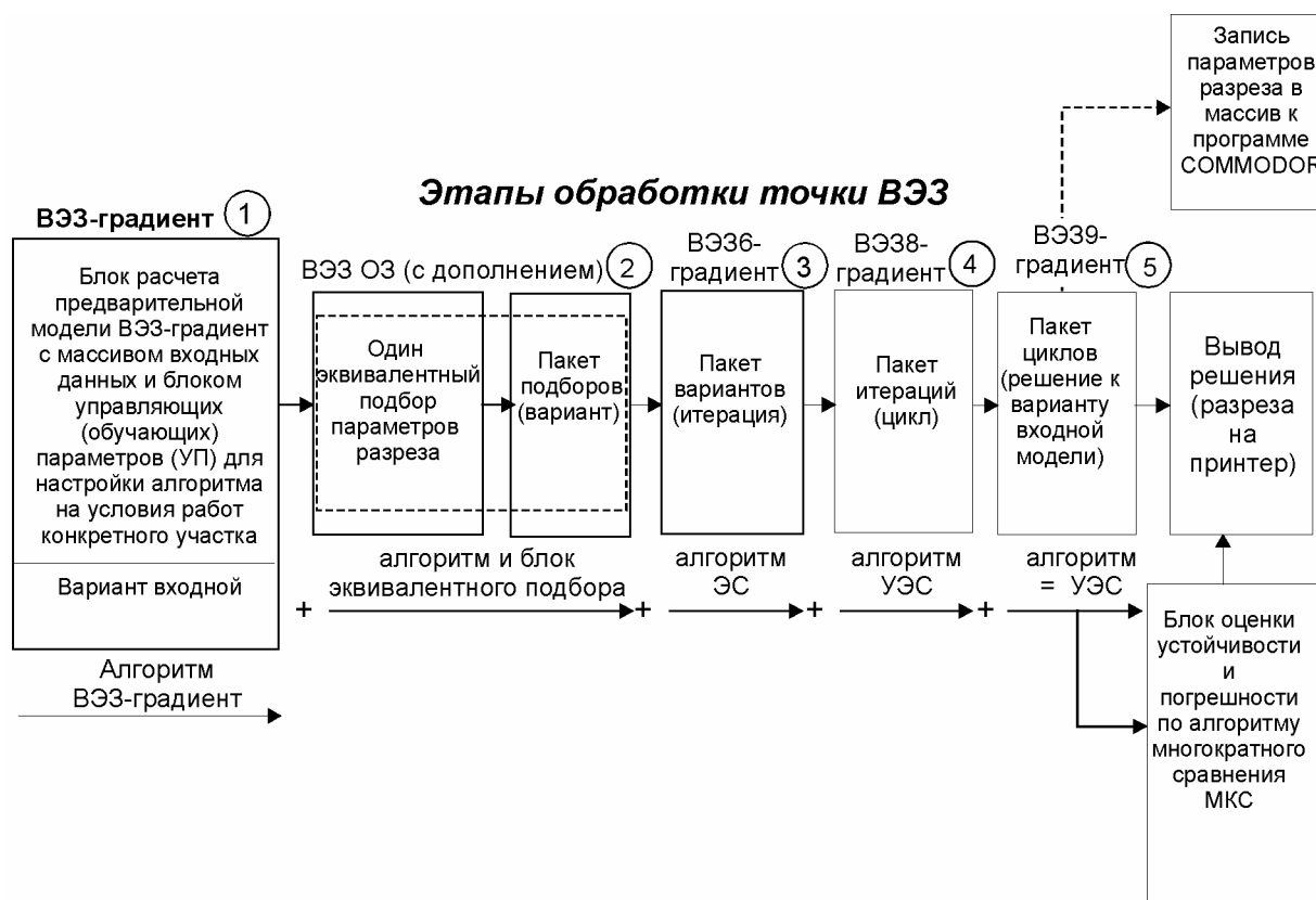
Блок-схема алгоритма УЭС1.
