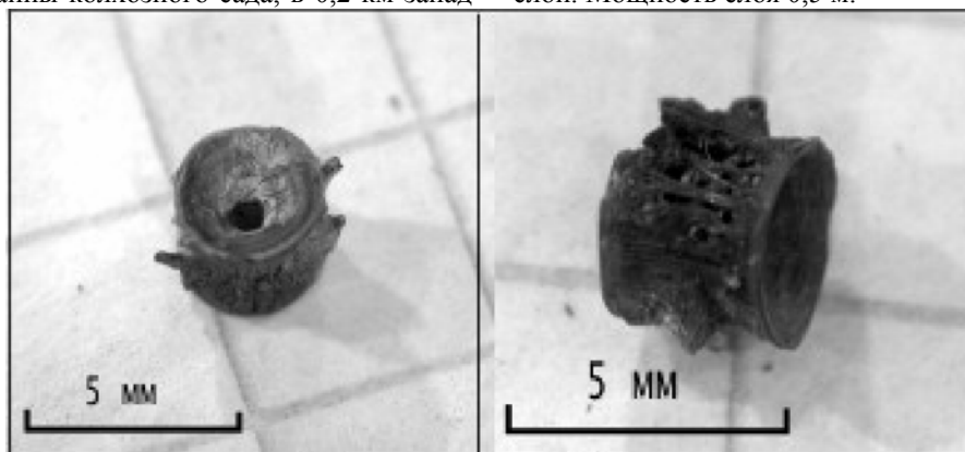
Рис. 2. Хвостовые позвонки Salmo sp.
