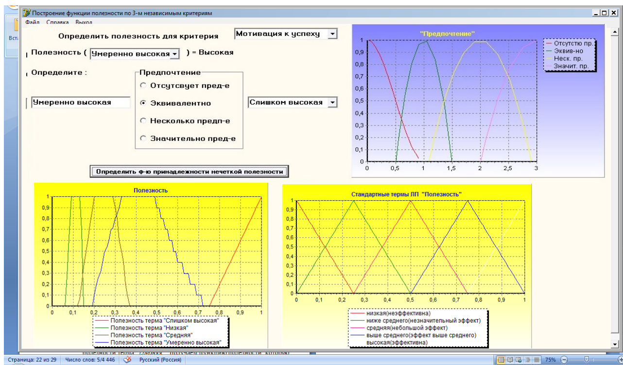
Рис. 4. Функции полезности термов критерия «Мотивация к успеху»
