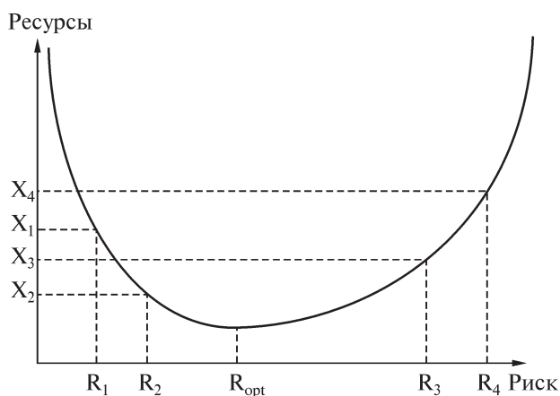
Рис. 1. Изокванта функции U(X,R)
