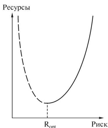
Рис. 3. Изокванта для катастрофического риска
