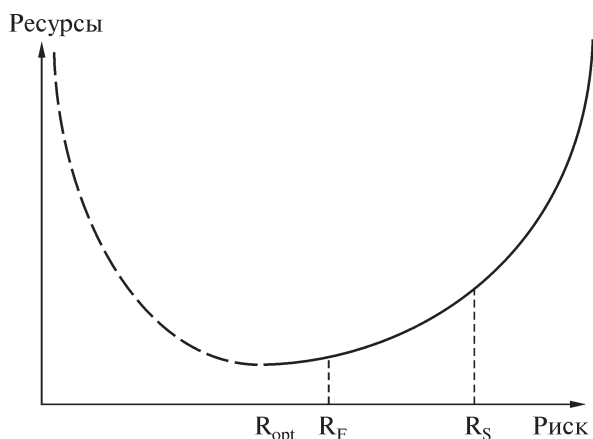
Рис. 2. Вид изокванты для систематического риска
